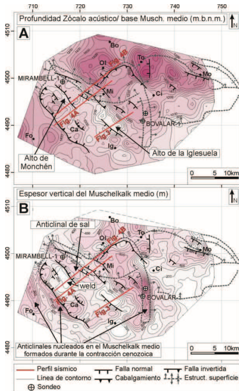
FIGURA 2. A: Mapa de contornos de la profundidad del zócalo acústico o base del Muschelkalk medio, en metros bajo el nivel del mar (m.b.n.m.). B: Mapa de isopacas del Muschelkalk medio.
