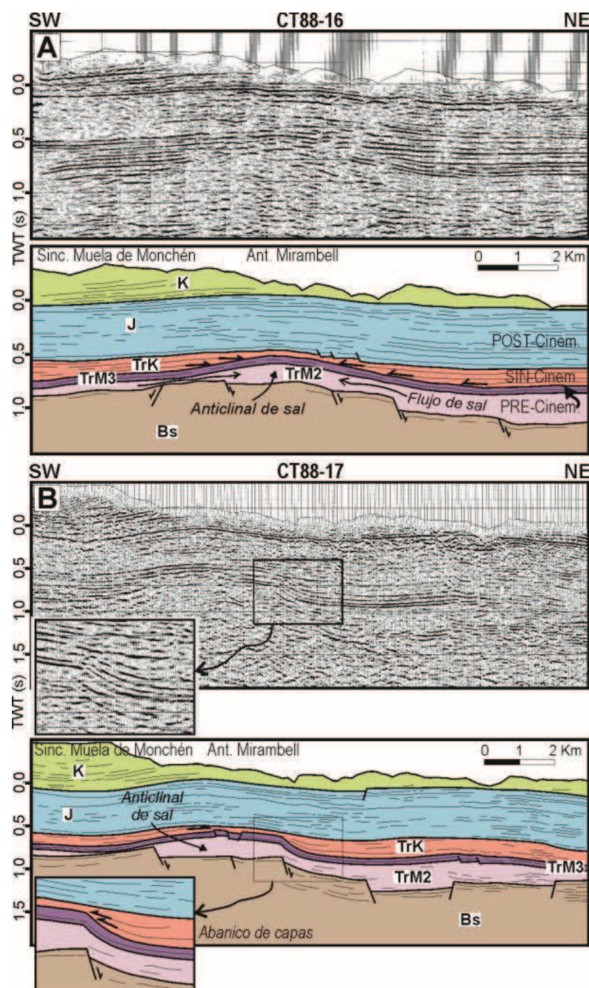
FIGURA 4. A: Perfil sísmico CT88-16 y su interpretación. Se muestra un anticlinal de sal de la facies Muschelkalk medio y los reflectores del Keuper en onlap sobre el Muschelkalk superior plegado por la acumulación de sal. Pre-, sin-, y post-cinemático se refieren al flujo de sal. B: Perfil sísmico CT88-17 y su interpretación. Se muestra un pliegue forzado del Muschelkalk superior sobre una falla de zócalo reactivada durante el depósito de la facies Keuper, que forma un abanico de capas sobre el pliegue. Ver localización en la Fig. 1.
