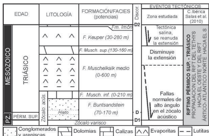
FIGURA 5. Esquema tectonoestratigráfico del Triásico en la parte central de la Cuenca del Maestrat.
