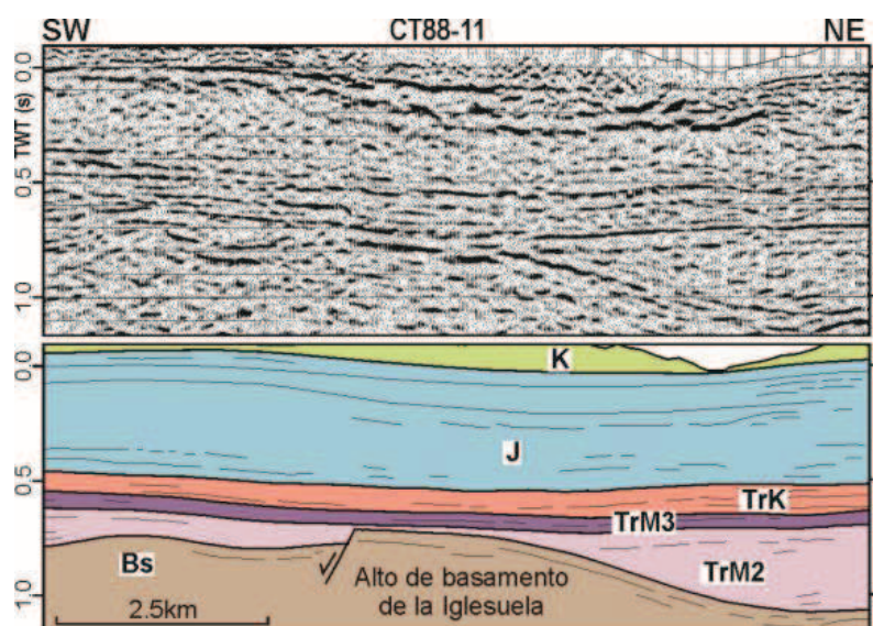
FIGURA 3. Perfil sísmico CT88-11 y su interpretación. Se muestran los cambios de espesor deposicionales de la facies Muschelkalk medio. Ver localización en la Fig. 1. Abreviaciones: K-Cretácico, J-Jurásico, TrK-Keuper, TrM3-Muschelkalk superior, TrM2-Muschelkalk medio, Bs-Zócalo acústico.
