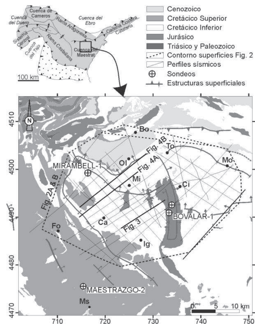
FIGURA 1. A: Mapa de situación de la zona de estudio, en la parte central de la Cuenca del Maestrat. En gris, áreas con zócalo involucrado; en punteado, áreas con sólo la cobertera involucrada. B: Mapa geológico simplificado de la zona de estudio y localización de los perfiles sísmicos y los sondeos analizados. Abreviaciones de localidades: Bo-Bordón, Ca-Cantavieja, Ci-Cinctorres, Fo-Fortanete, Ig-Iglesuela del Cid, Mi-Mirambell, Mo-Morella, Ms-Mosqueruela, Ol-Olocau del Rey.
