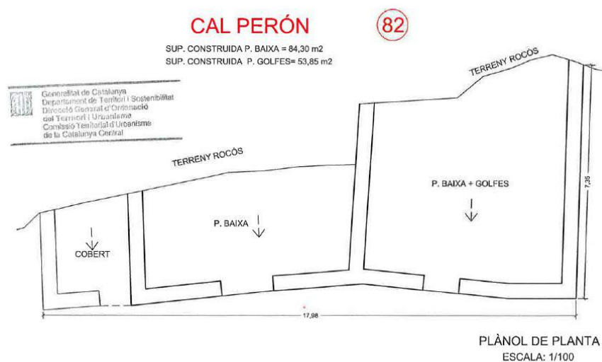
Fig.E 6: Planta de Cal Perón, on es pot observar l'adossament a la roca. Font: Pla Especial de Peguera
