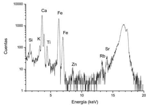
2. Muestra procedente de la Cova la Sarsa (N.7).
