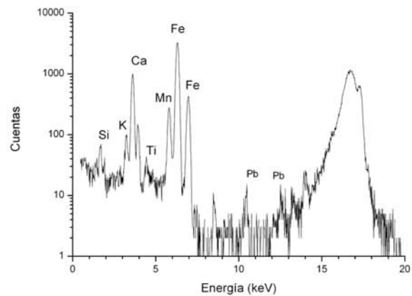
3. Muestra procedente de la Cova Fosca (N.8).
