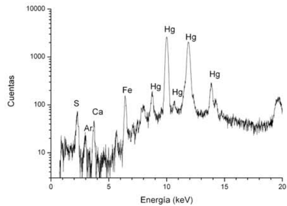
1. Muestra procedente de la Cova de l'Or (N.6).
