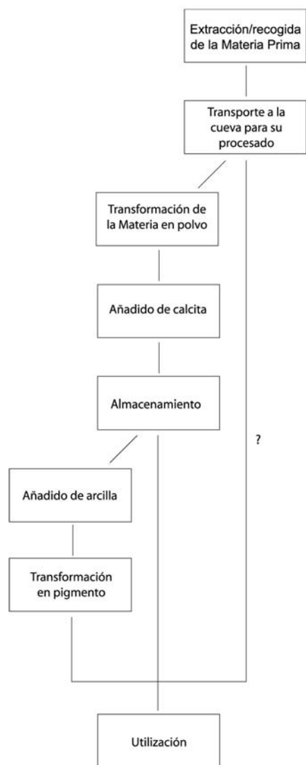
Fig. 3. Propuesta de cadena operativa para la producción y utilización de colorante en la Cova de l'Or
