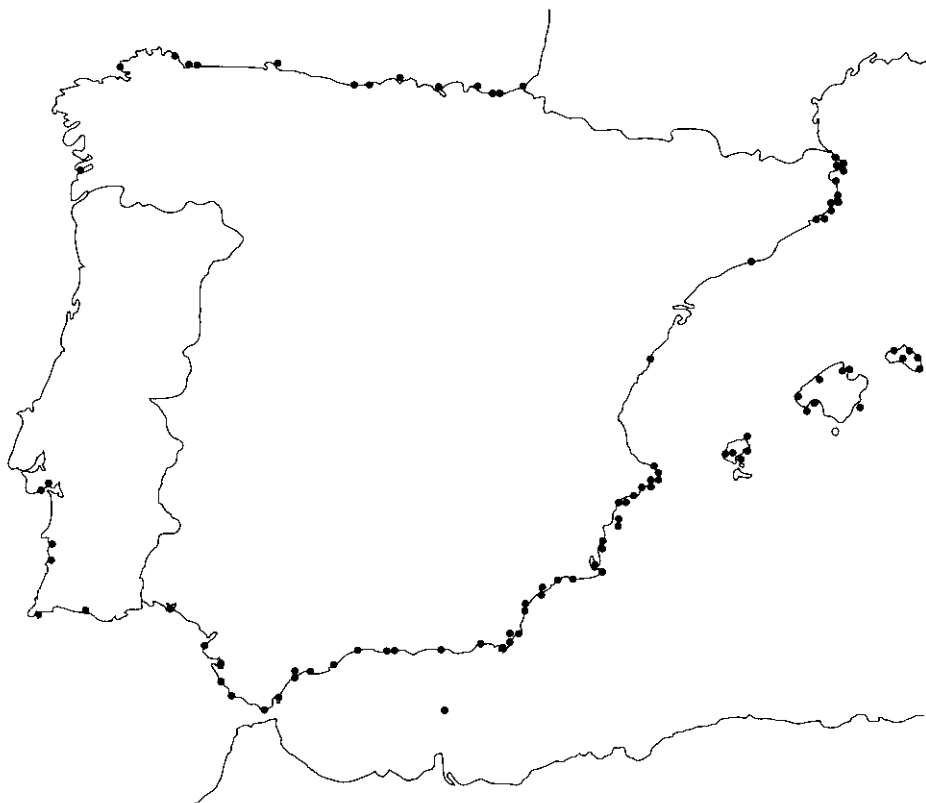
Mapa 2.—Distribución de Padina pavonica en la Península Ibérica e Islas Baleares.
