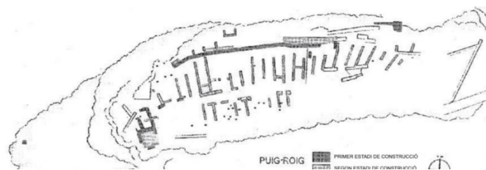
Fig. 2 Planta del Puig Roig (Rafel, N., 2008, 258)
