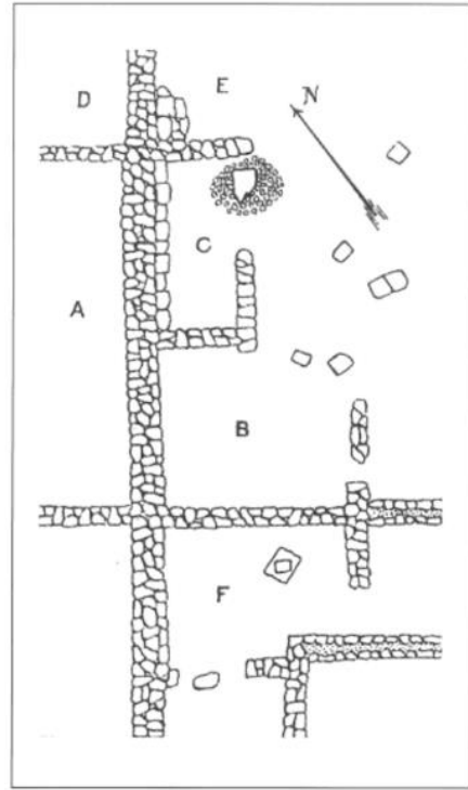
Fig. 8 Planta dels recintes excavats per Vilaseca al Calvari del Molar (Rafel, N., et al. 2001)
