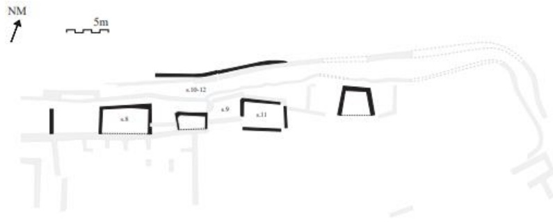
Fig. 9 Planta Fase 1 del Calvari del Molar (Edifici pròpia)
