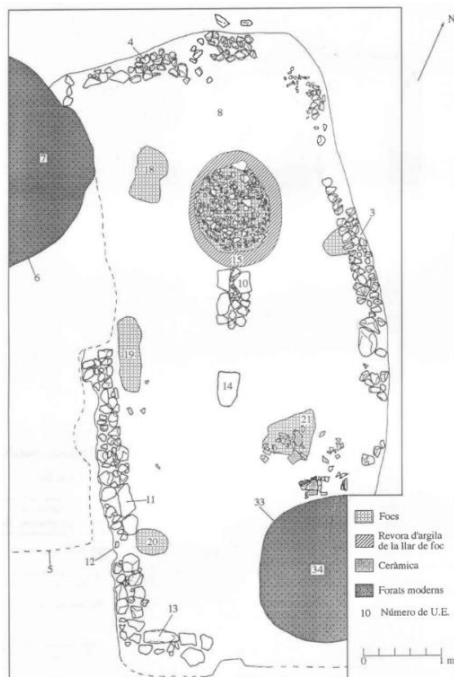
Fig. 1 Planta de la darrera fase del Barranc de Sant Antoni (Noguera, J., 1998, 105)
