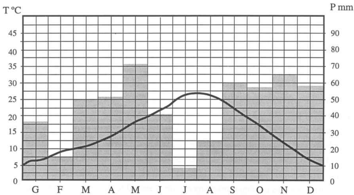
Diagrama ombrotèrmic de l'estació de Móra d'Ebre. La temperatura mitjana anual oscil·la entre els 14° i els 16°C. A uns estius calorosos i eixuts segueixen unes tardors suaus i plujoses, uns hiverns temperats i més aviat eixuts, i unes primaveres també suaus i plujoses ( Geografia Comarcal de Catalunya , 1993: 400).
