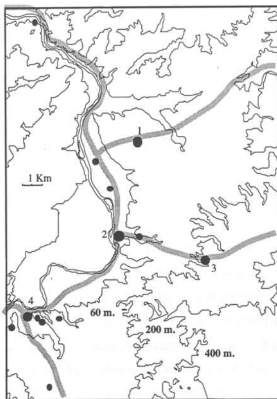
Localització dels assentaments altimperials sobre la xarxa viària de la foia de Móra, comunicant amb el Priorat (núm. 1, les Planes) i amb la costa a través de la Serra de Tivissa (núm. 3, l'Aumedina i núm. 2, Mas de Molló 2) i la plana de Burgar (núm. 4, les Pedres).
