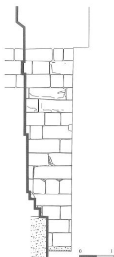
Figura 25. Alçat del mur andalusí documentat a la sala 4 realitzada a l'interior de la Seu Vella (Lorient, 1997: 82).
