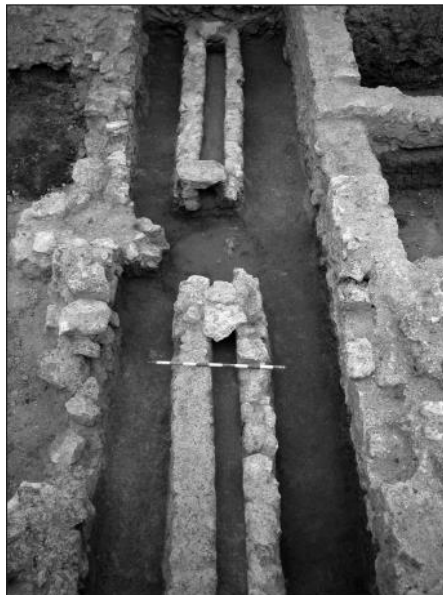
Figura 14. Fotografia que mostra un tram de la xarxa de clavegueram del c/Montcada (Bea et al. , 2011: 500).
