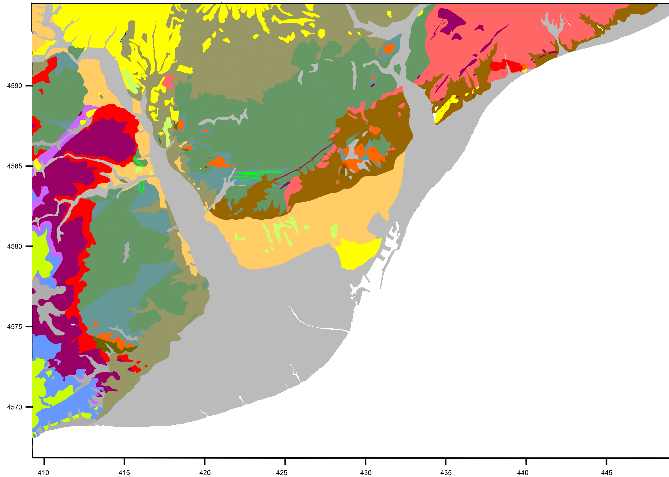
Figura 2. Mapa Geológico de Barcelona y alrededores (modificado de las cartografías 1:50.000 de IGME 1975 a, b, c)
