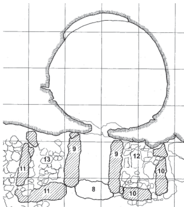
Fig. 6: Plànol de la planta de l'hipogeu de planta simple de Sant Tomás (GUERRERO et al., 2006a)
