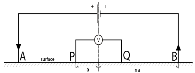
Fig. 1: Schlumberger array [1].
