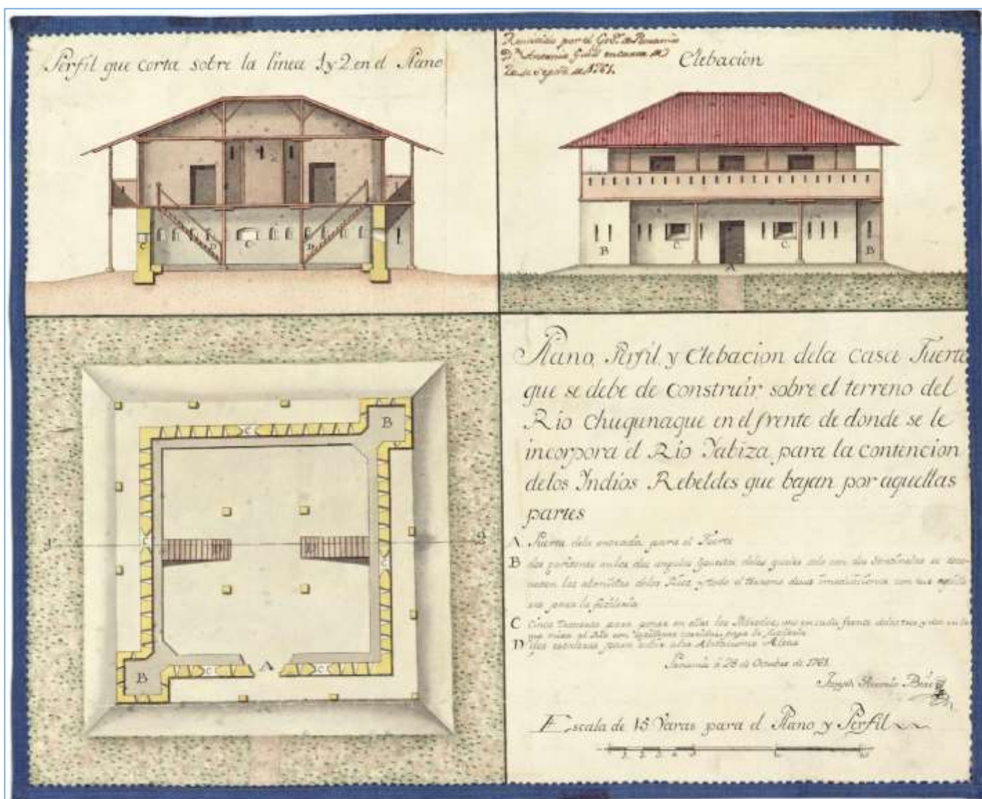
(Mapa 20) Plano, Perfil y Elevación de la casa Fuerte que se debe de construir sobre el terreno del Río Chucunaque en el frente de donde se le incorpora el Río Yaviza, para contención de los Indios Rebeldes que bajan por aquellas partes. 1761. Fuente: CCGE (BVD) Ar. J-T.4-C.4-42
