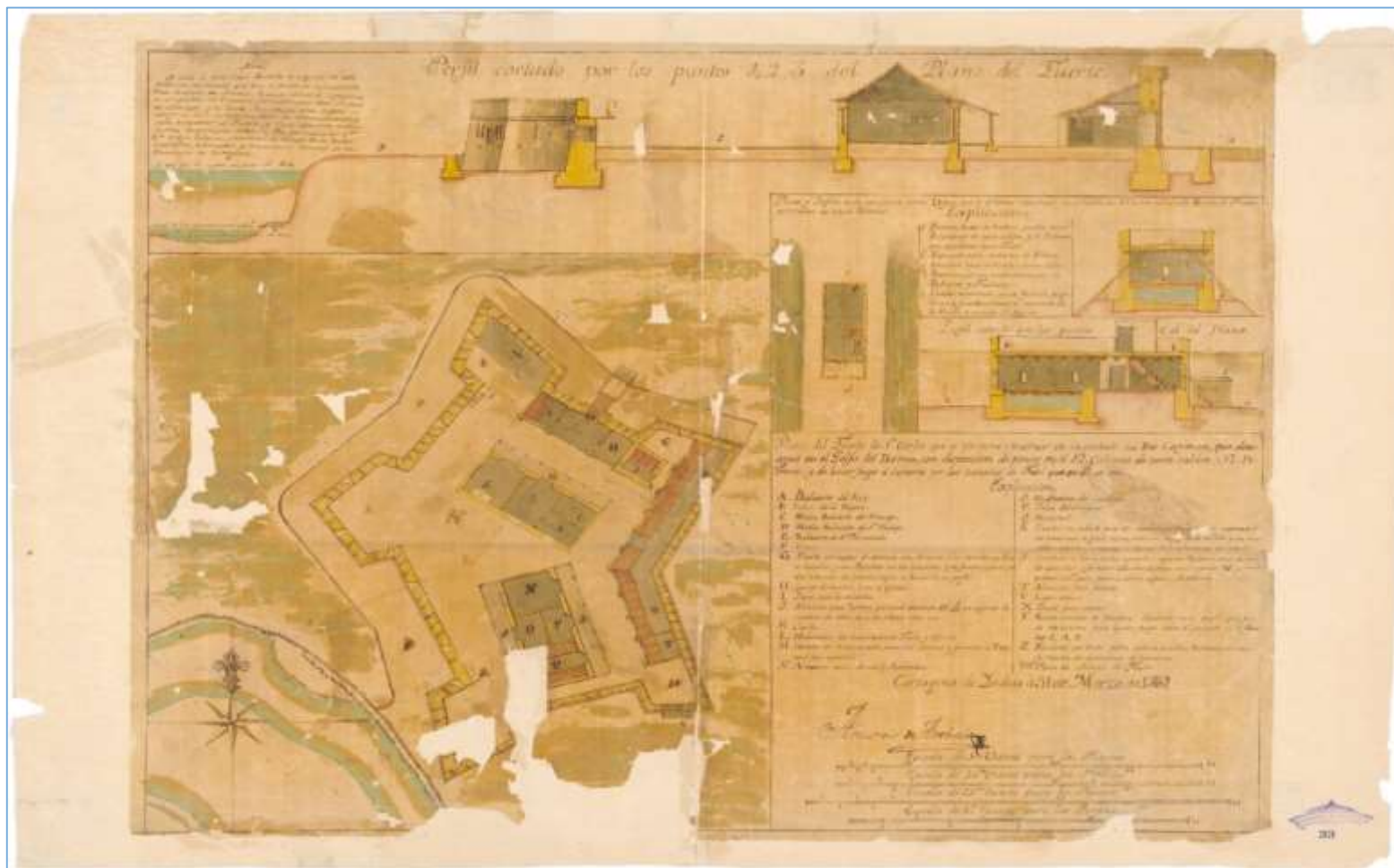
(Mapa 23) Plano del Fuerte de Sn. Carlos que se propone construir en un costado del Río Caimán, que desagua en el Golfo del Darién: con disposición de poner en él 12 cañones de corto calibre y 12 Pedreros y de hacer fuego a cubierto por las troneras de Fusil que en él se ven. Fuente: CCGE Ar. J-T.7-C.3-99
