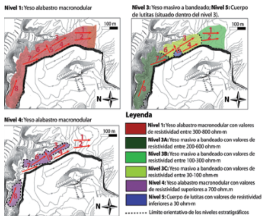
Figura 7: Cartografía de la superficie del techo de los diferentes niveles estratigráficos definidos en el frente de cantera (Área 1, Fig. 4). 1 a 8: perfiles tomográficos. Niveles 3A, 3B, 3C: el nivel 3 masivo-bandeado se ha dividido en función de sus resistividades; estos valores se pueden correlacionar con la pureza en yeso de los cuerpos, siendo los más resistivos los más ricos en yeso.
