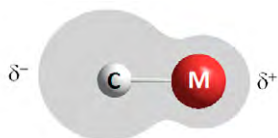
Figura 1. Representació de la polaritat d'un enllaç carboni-metall.
