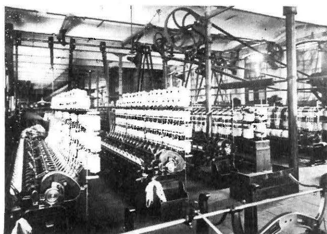
Fot. 12. Correspon a la fàbrica Garriga. Aquestes màquines són les metxeres, fan el que se'n diu falsa torsió, és a dir, estiren el fil sense arribar a fer la torsió pròpia del filat.
