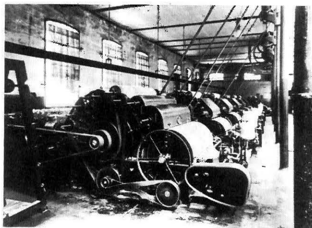
Fot. 8. Fotografia de la filatura de la fàbrica "Garriga". Tenim unes cardes. En aquestes màquines la llana es neteja de totes les impureses que encara resten després del rentat. També estiren la fibra i la fan més esponjosa. Comencen ja a preparar la fibra per a ser filada.
