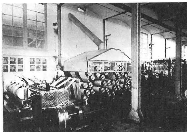
Fot. 9. Fotografia de "La Lanera Española". Continúa la preparació del fil. Aquí torna a ser rentada i pentinada. Fixeu-vos que en aquest cas el que es renta i es pentina ja és la fibra estirada. Abans havíem rentat els flocs de llana.
