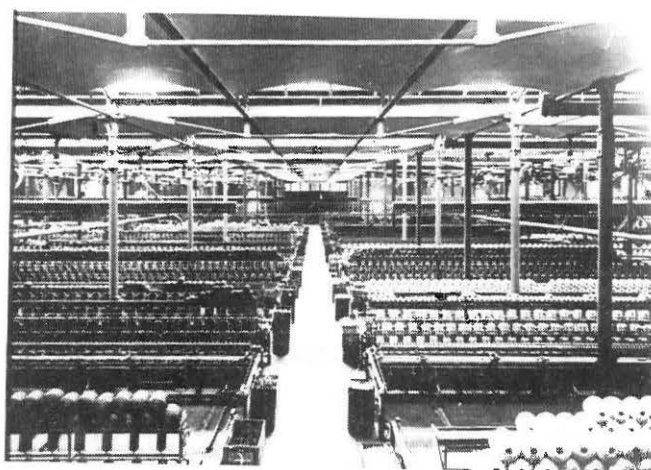
Fot. 14. Fotografia de "Can Quadras i Prim". També es una sala de contínues per filar. Aquestes màquines s'anomenen "selfactines" i tenen la mateixa funció que les que hem vist a la fotografia nº 13.
