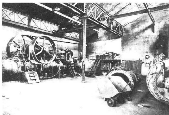
Fot. 3. Aquí tens una perspectiva general de la sala on estava instal·lat un vapor. Ja saps que els vapors servien per a fer funcionar les màquines de les fàbriques. Des d'aquí aquesta màquina podia produir l'energia suficient per al funcionament de les diferents naus.
