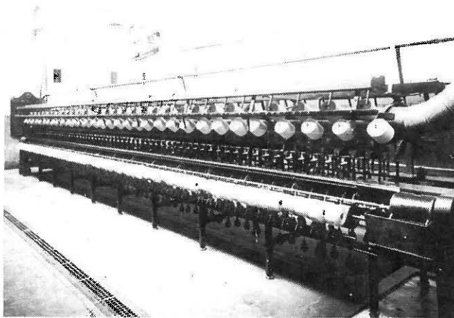
Fot. 16. Fotografia de "Can Carol". Aquí es fan les bobines: són les màquines bobinadores. S'acaba el filat, el fil ja està llest per a començar el procés del tissatge.
