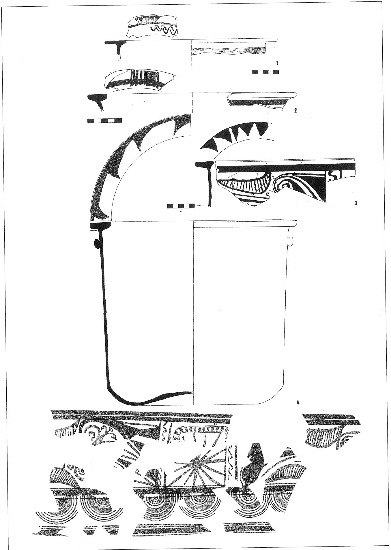
Fig. 12. Forma 4.3. 1. Plaça de Sant Joan (Lleida) (segons JUNYENT, PÉREZ 1995, 227); 2. La Paeria (Lleida); 3. Camp Primer (Guissona) (segons GUITART et al. 1998, fig. 13); 4. Missatges (Tàrraga) (segons GARCÉS, SAULA 1996, 43-44).
