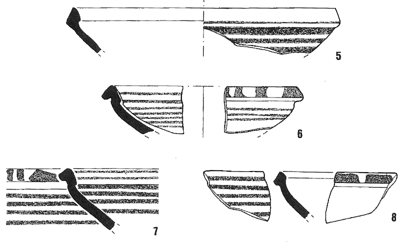
Fig. 8. Formes 2.7. a 2.8. 1-2. Raimat (Lleida) (segons GARCÉS 1988, 39). 3-7. Antic Portal de Magdalena (Lleida).
