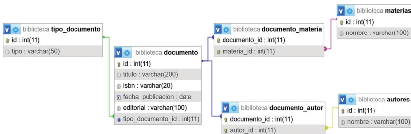
Figura 41. Ejemplo relaciones y atributos
