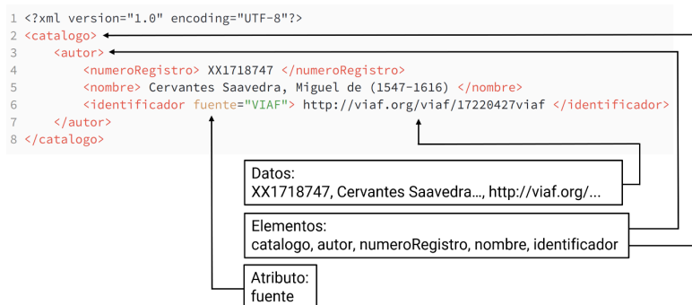
Figura 48. Componentes de un documento XML
