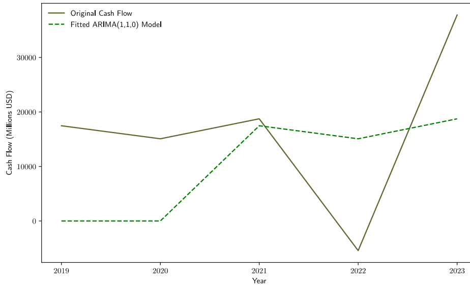
Figure 9. ARIMA(1,1,0) Model Fit for Électricité de France. Source: Own Preparation.
