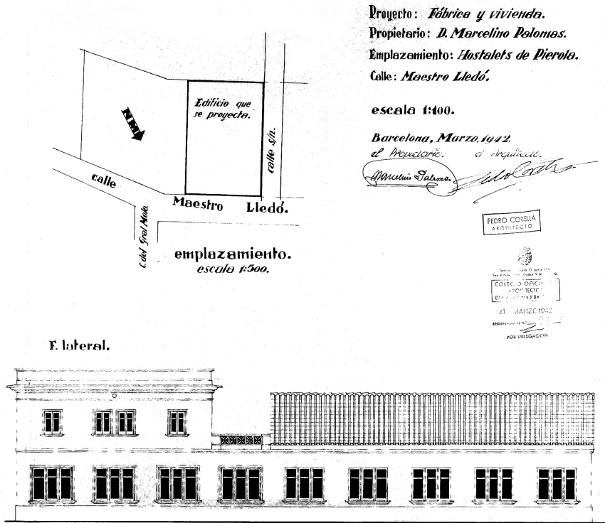
Figura 2. Emplaçament i façana lateral de la nova fàbrica de Marcel·lí Palomas (1942)
