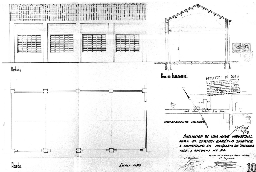
Figura 3. Projecte presentat per a la sol·licitud de llicència municipal d'obres per a la construcció de la fàbrica de Textil ISAGAR SL (1959)
