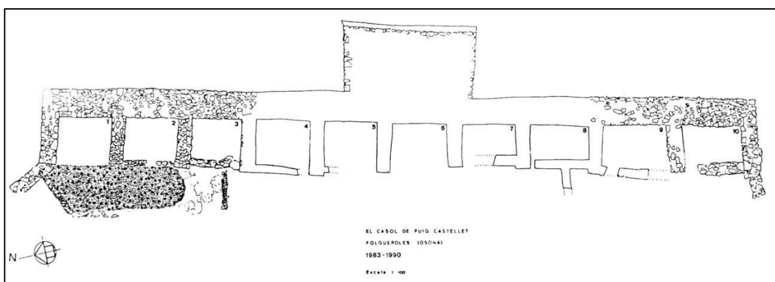
Figura 5: Planimetria general de la fortalesa del Casol de Puigcastellet. (Dibuix: Elisabet Huntingford)
