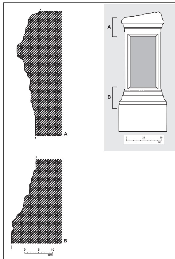
Figura 4. Perfil y croquis a escala del ara (Dibujo: Ramón Álvarez).
