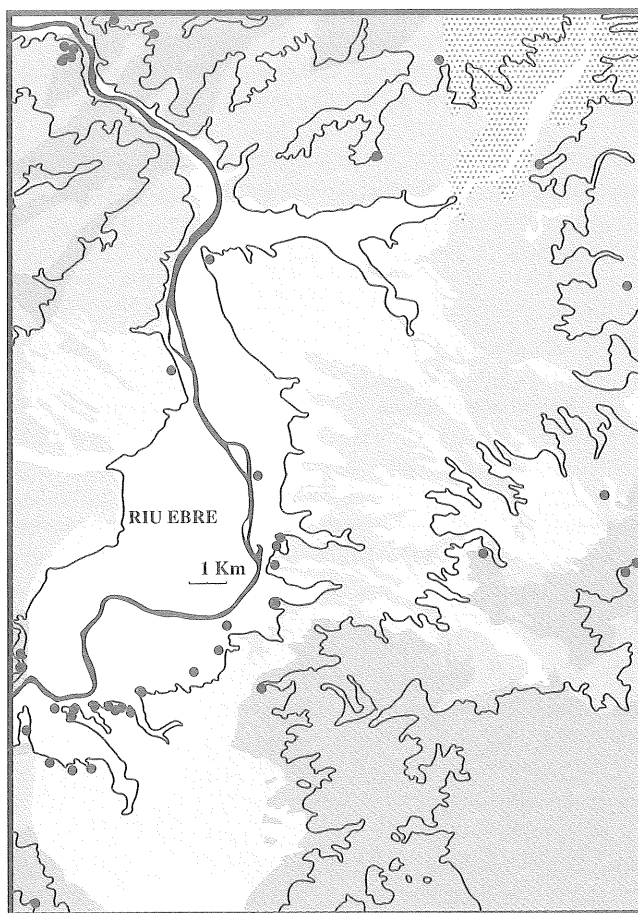
Figura 2. Mapa geològic de la cubeta de Móra, amb la localització dels jaciments mencionats en el text.
