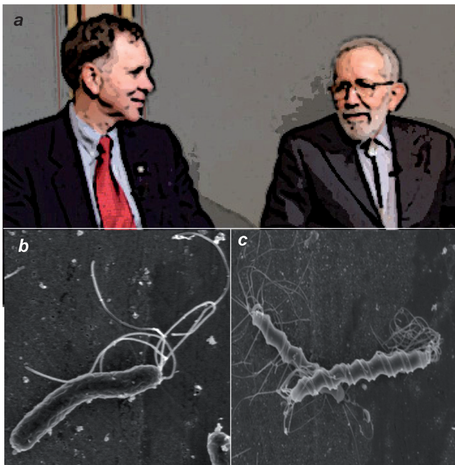
Figura 3 a) Barry J. Marshall (esquerra) i J. Robin Warren (dreta), el desembre de 2005 (dibuix a partir d'una foto). b) Micrografia amb el microscopi electrònic de rastreig d' Helicobacter pylori aïllat de l'epiteli gàstric humà. S'aprecia la forma corbada del bacteri. c) Micrografia amb el microscopi electrònic de rastreig d' Helicobacter felis aïllat de la mucosa gàstrica d'un gat. Micrografies de Lucinda Thompson, publicades a Int. Microbiol. , 8: 231-234, amb permís de la revista.
