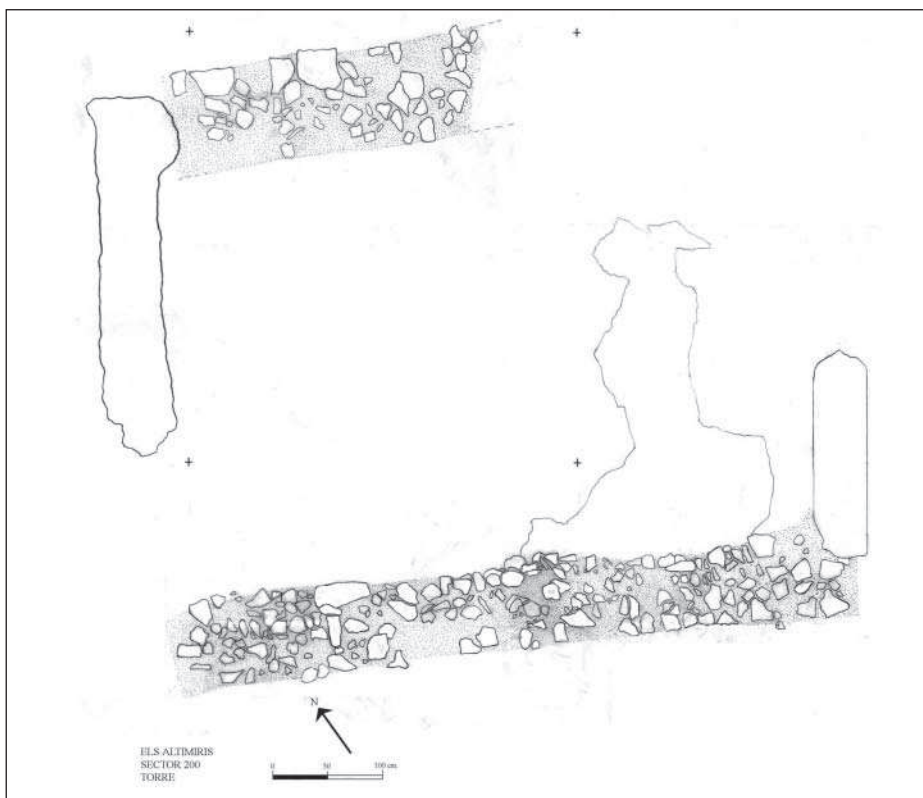
Figura 4. Planta de la torre on es veu el fragment de paviment conservat i els 4 murs de tancament parcialment excavats
