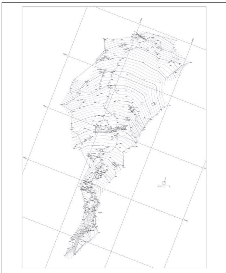
Figura 1. Aixecament topogràfic del jaciment dels Altimiris. S'hi pot observar la forma triangular del jaciment que queda delimitat per cingleres a dreta i esquerra. A baix, el pas de Santa Cecília i a dalt, el costat més ample del triangle que creiem que queda delimitat per un mur de tancament o muralla. Al centre, l'església i al seu costat, els dos fons de cabana excavats. La torre es troba situada just abans de la part més estreta del triangle a la dreta
