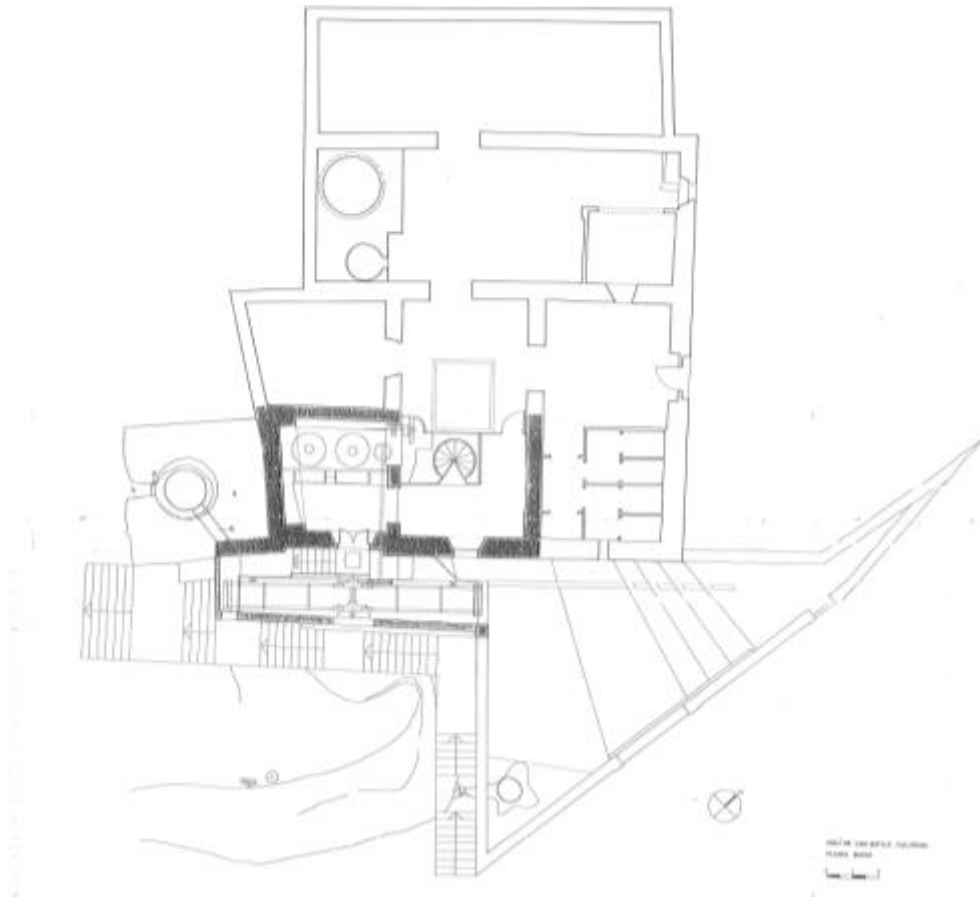
Fig. 19: Planta de la masia. He posat aquest dibuix perquè es veu ben representada la bassa, que queda tallada a la secció transversal. Just a l'encaix entre el pou i la bassa es troba la roda vertical, que funciona per acció de gravetat.
