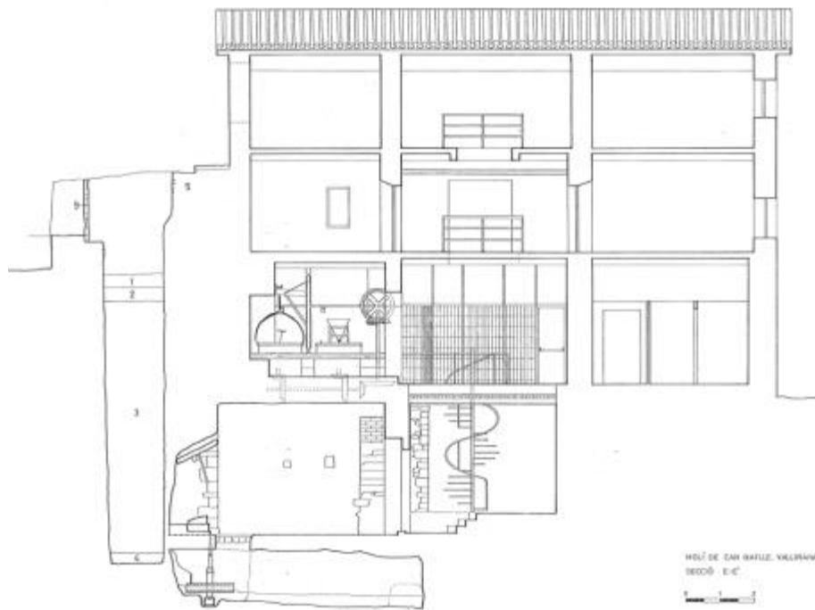
Fig. 18: Secció transversal de la Masia Can Batlle a l'actualitat, realitzada després de la intervenció arqueològica. El que fa interessant, és la bona conservació del pou, l'obrador i la sala de les moles.
