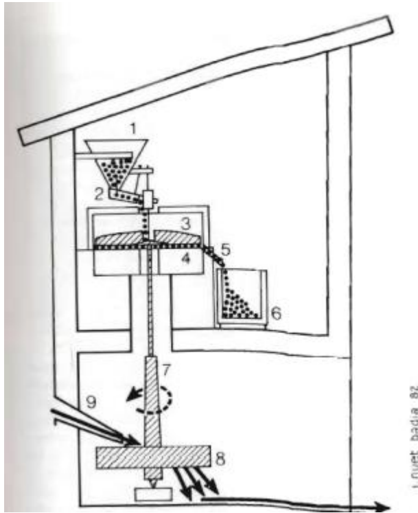
Fig. 2: Esquema d'un molí fariner de roda horitzontal. Il·lustra el funcionament i les parts dels mecanismes (Bolòs; Nuet, 1983:31).
