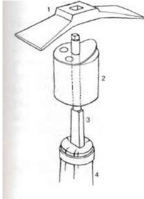
Fig. 1: Esquema de la nadilla i l'arbre. Exemple d'un molí fariner de roda horitzontal (Bolòs; Nuet, 1983:31).
