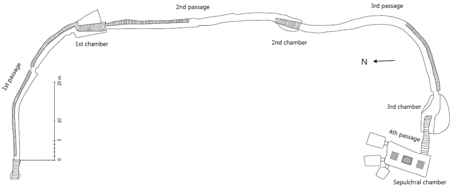
Figura 23: Planimetria de KV 20. Font: WILLOCKX (2011a).
