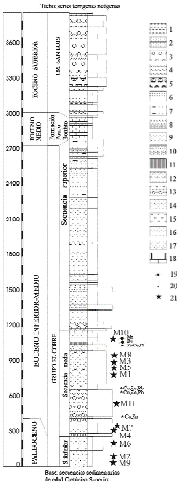
Figura 2. Localización de las muestras estudiadas en la columna geológica generalizada de las series del Paleógeno desarrolladas en la parte oriental de la Sierra Maestra, a través del Yacimiento "El Cobre": 1-limolitas, 2-areniscas calcáreas, 3-conglomerados, 4-microconglomerados, 5-conglomerados calcáreos, 6-areniscas polimícticas, 7-areniscas tobáceas, 8-rocas piroclásticas calcáreas, 9-rocas piroclásticas intermedias a ácidas, 10- aglomerados, 11-cuerpos estratiformes de anhidrita, 12-brecha volcánica con predominio de fragmentos de tamaño < 15 mm y abundantes intercalaciones de areniscas y rocas piroclásticas, 13-brecha volcánica con fragmentos de tamaño generalmente > 15 mm y pocas intercalaciones de areniscas y rocas piroclásticas, 14-andesita basáltica, 15-andesitas, 16-andesita-dacita, 17-rocas piroclásticas intermedias a básicas, 18-calizas, 19- mineralización estratiforme, 20- mineralización estratoligada, 21- localización de las muestras de rocas volcánicas estudiadas.
