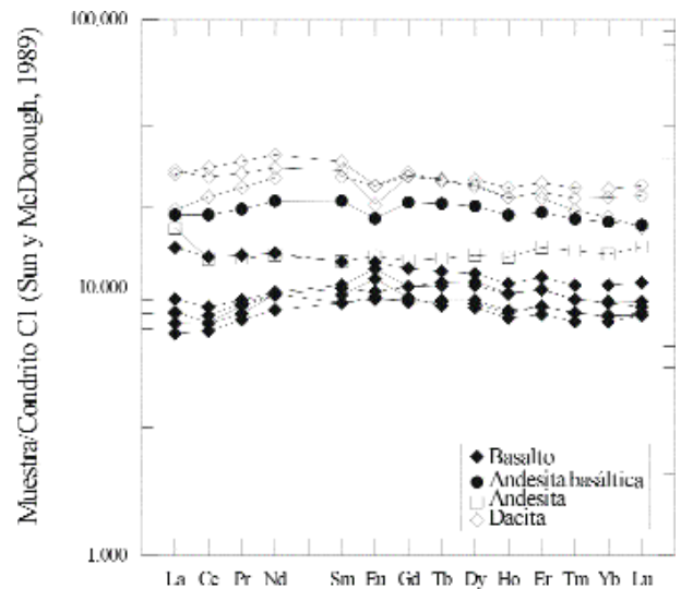
Figura 8. Diagrama de REE, normalizados a los valores condriticos, de las rocas volcánicas de las series inferior y media del Grupo El Cobre en la Sierra Maestra.
