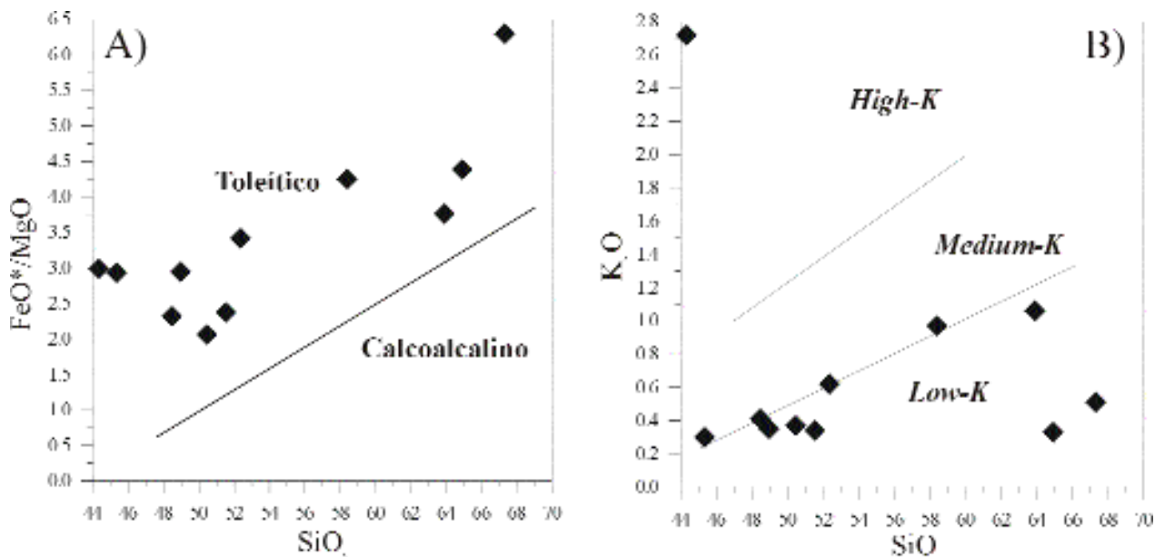
Figura 7. A) Variación del hierro total (expresado como FeO^*/MgO ) frente a SiO_2 en las rocas volcánicas presentes en las series inferior y media del Grupo El Cobre en la Sierra Maestra. La línea de discriminación de los campos tholeiíticos y calcoalcálico es trazada a partir de Miyashiro (1974). B) Variación del K_2O frente a SiO_2 en las mismas rocas. Los campos son tomados de Gil (1981).
