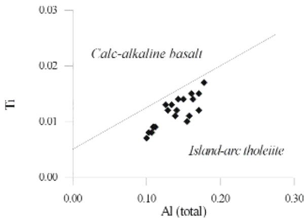
Figura 10. Variación de Ti con respecto a Al total en fenocristales de clinopiroxenos en las rocas volcánicas (basaltos y andesitas basálticas) de las series inferior y media del Grupo El Cobre en la Sierra Maestra. Nótese como todas las muestras caen dentro del campo de las tholeiitas de arcos de isla definido por Leterrier et al. (1982).
