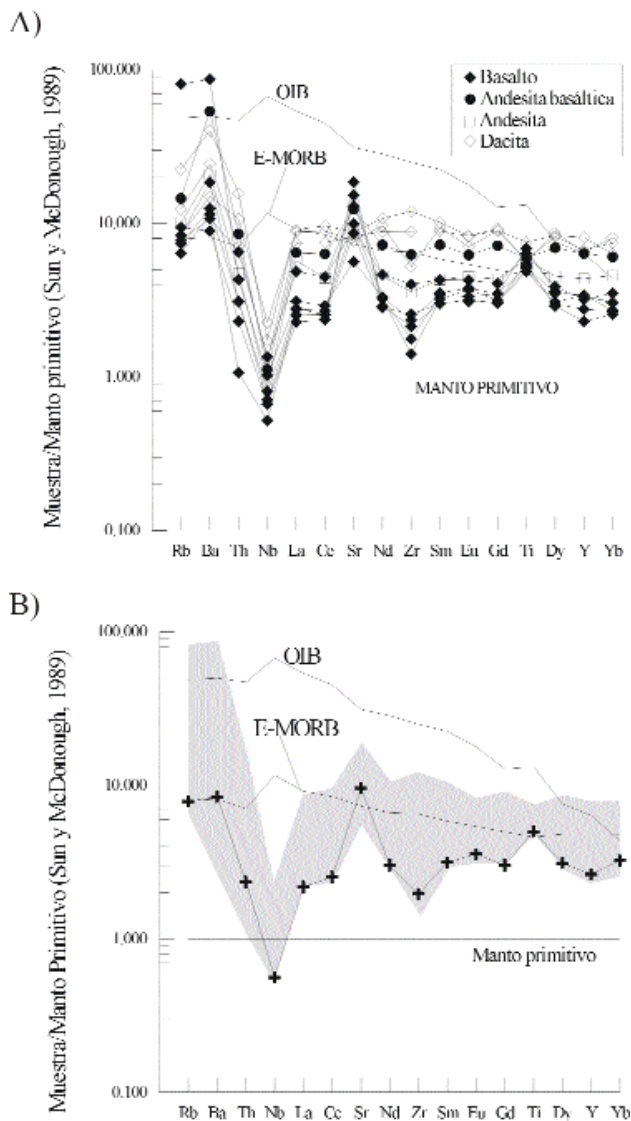
Figura 9. A) Diagrama de elementos trazas, normalizados al manto primitivo, de las rocas volcánicas de las series inferior y media del Grupo El Cobre en la Sierra Maestra. B) Comparación del patrón de distribución de los elementos trazas de las mismas rocas (zona sombreada) con el arco de Kermadec (cruces) en Pacífico SW. Los valores del manto primitivo, OIB y E-MORB pertenecen a Sun y McDonough (1989). Los datos del arco de Kermadec son tomados de Smith et al. (1997).
