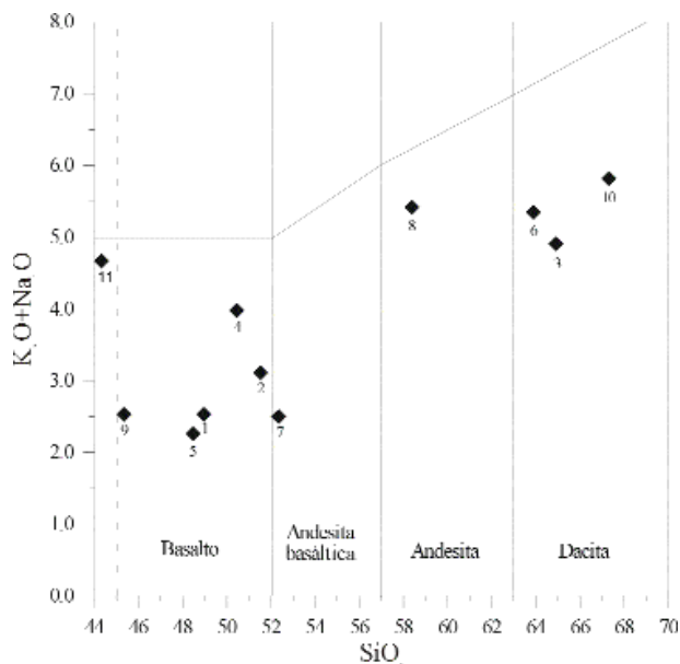
Figura 6. Álcali total ( \text{Na}_2\text{O} + \text{K}_2\text{O} ) frente a \text{SiO}_2 (TAS) en las rocas volcánicas presentes en las series inferior y media del Grupo El Cobre en la Sierra Maestra. Los campos son de Le Bas et al. (1986).
