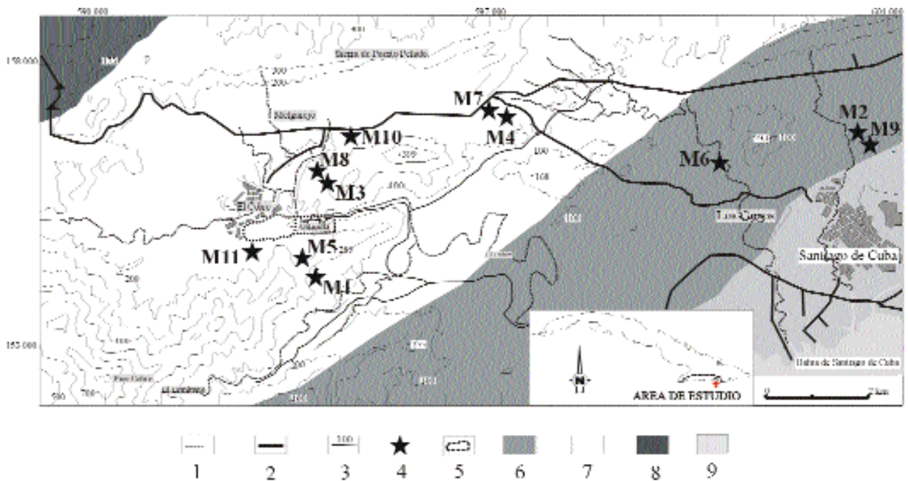
Figura 3. Mapa esquemático de la Sierra Maestra con la ubicación de las muestras de rocas volcánicas estudiadas. 1- Red fluvial, 2- carretera, 3- curvas de nivel, 4- localización de las muestras volcánicas estudiadas, 5- contorno de la corta del Yacimiento “El Cobre”, 6- parte inferior de las series del Grupo El Cobre, 7- parte media de las series del Grupo El Cobre, 8- parte superior de las series del Grupo El Cobre, 9- materiales terrígenos y carbonatados de Cuenca de Santiago.
