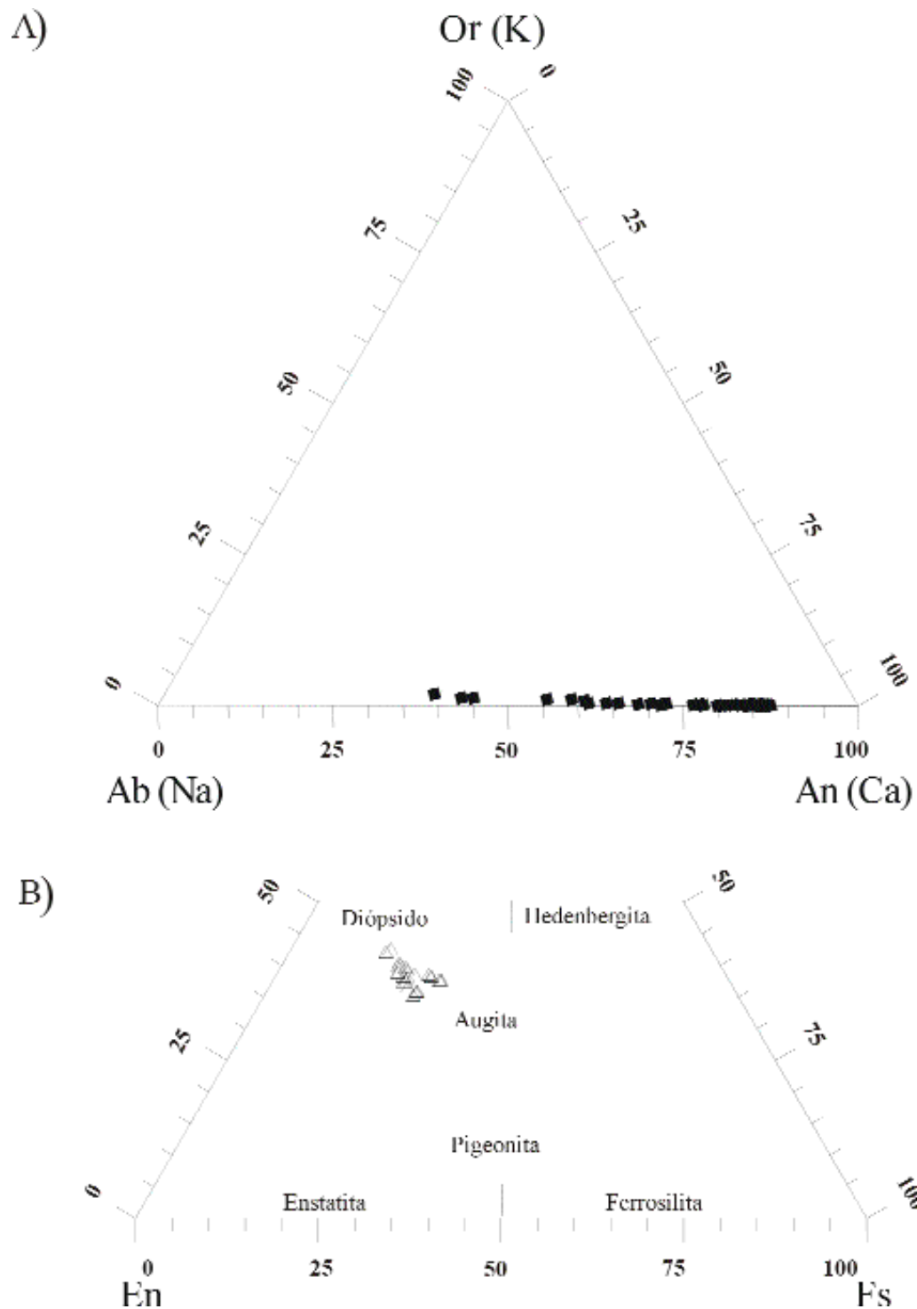
Figura 5. Composición de los fenocristales de plagioclasas (A) y de los de clinopiroxenos (B) presentes en las rocas volcánicas de las series inferior y media del Grupo El Cobre en la Sierra Maestra.
