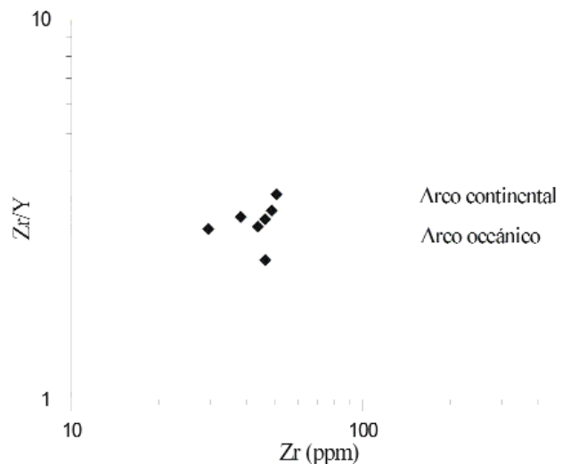
Figura 11. Variación de la relación Zr/Y con respecto a Zr en las rocas volcánicas (basaltos y andesitas basálticas) de las series inferior y media del Grupo El Cobre en la Sierra Maestra. Los campos de los basaltos de arco oceánico y de arco continental son de Pearce (1983).
