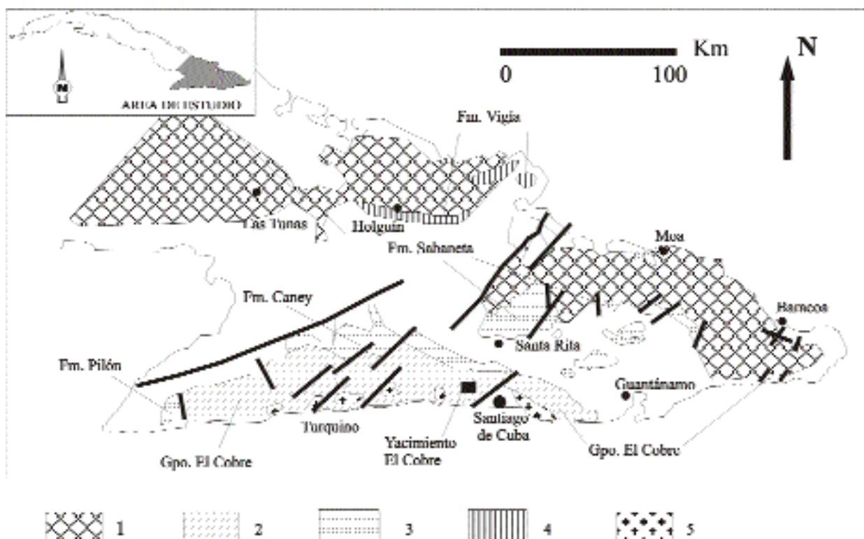
Figura 1. Grandes unidades en el Paleógeno de Cuba Oriental (adaptado de Iturralde-Vinent, 1996). 1) Basamento del arco. Rocas del arco volcánico Daniense-Eoceno Inferior: 2) Flujos de basaltos a dacitas, con rocas piroclásticas, grauwacas y calizas; 3) Rocas piroclásticas con calizas, margas, y grauwacas; 4) Calizas, margas, rocas piroclásticas y algunas intercalaciones de grauwacas; 5) Rocas plutónicas eocenas.
