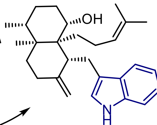
anominina
