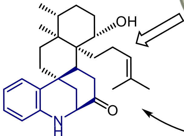
aspernomina
