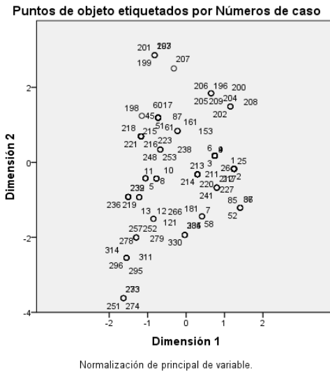
Figura II: Diagrama de dispersión de los objetos en torno a un promedio
