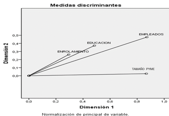
Figura I: Asociación de las variables originales con las dimensiones
