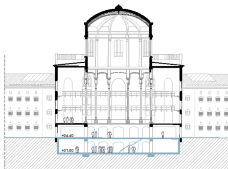
Secció Panòptic Central
