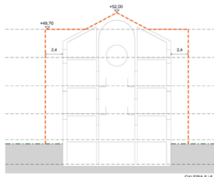
Secció A
