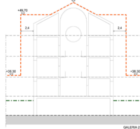
Secció C
