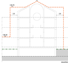
Secció D
