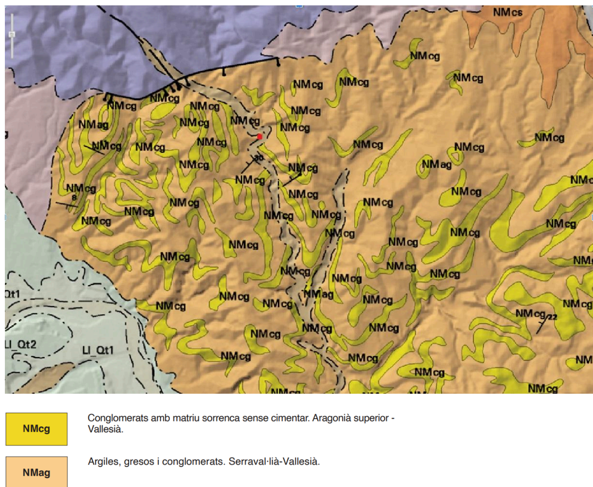
FIGURA 3. Extret del Mapa Geològic de Catalunya 1:250.000 (ICGC). El punt vermell indica el meandre de Sant Jaume.
