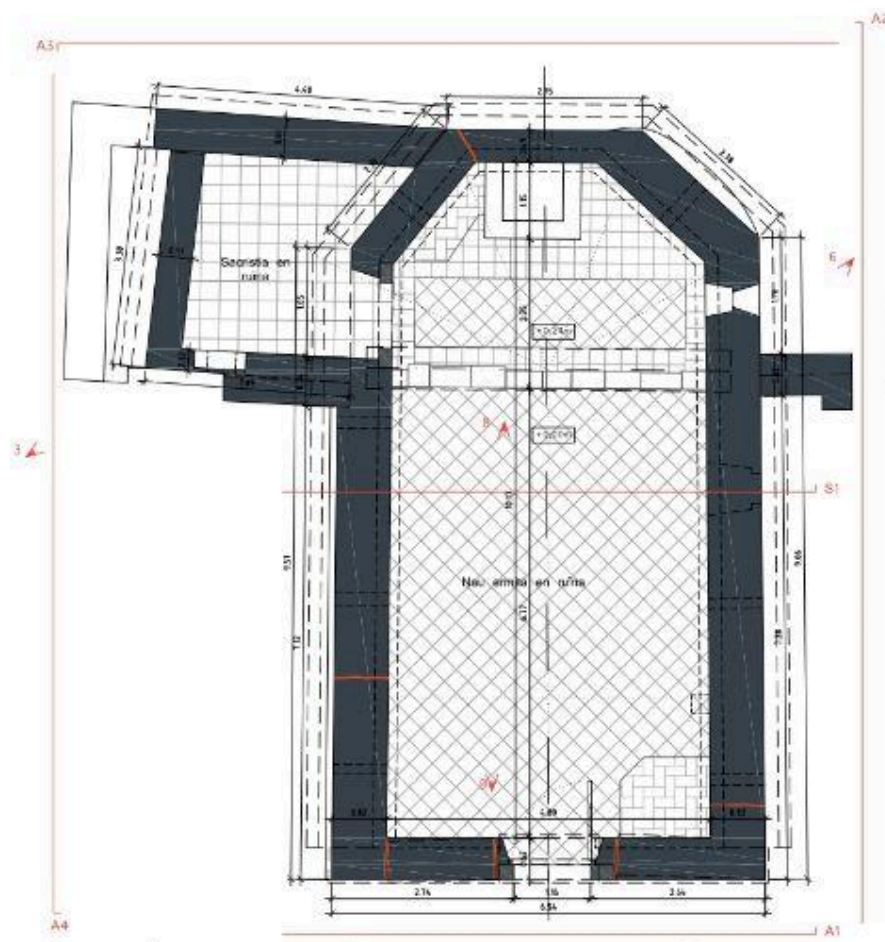
Plànols 1/50 de la capella; a l'esquerra de la planta i a la dreta de la secció central de la nau (cortesia d'Antoni Torrent).
