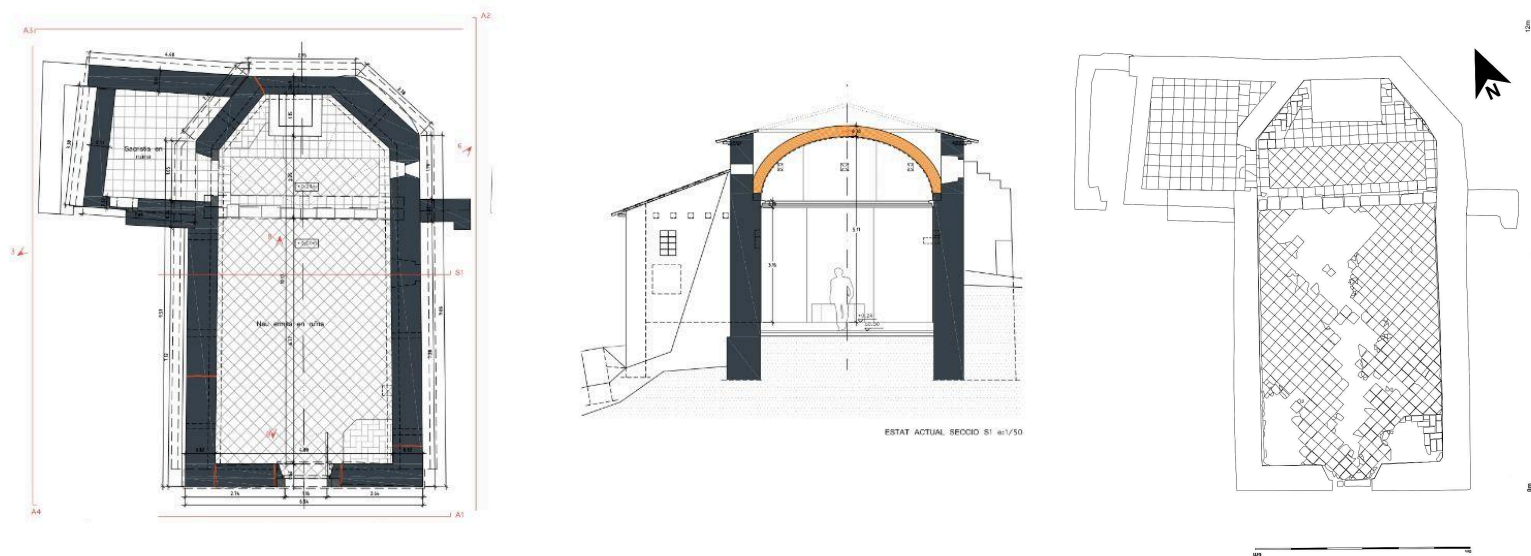
FIGURA 30. Plànols d'alçats i planta de la capella (més informació a l'Annex 7.1).
