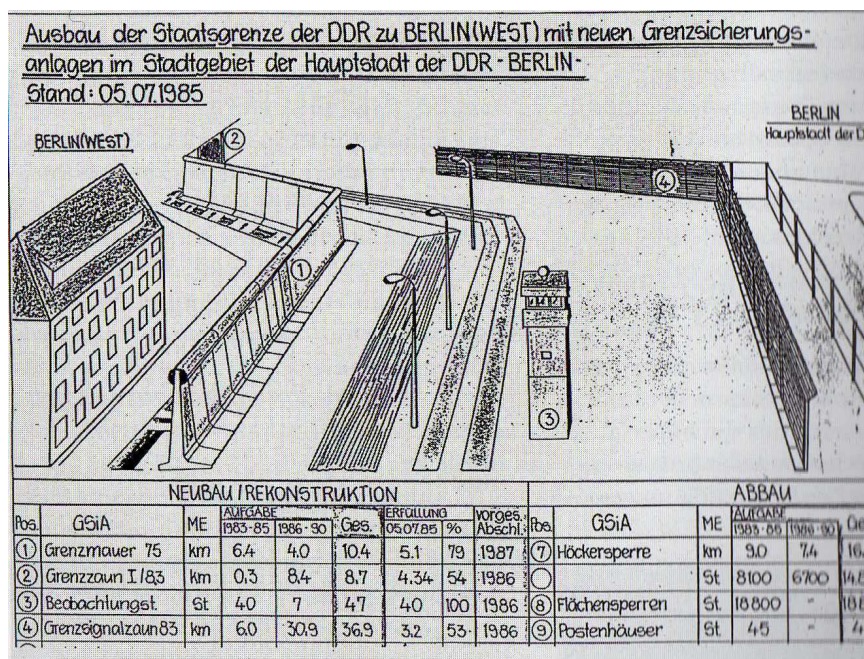
Fig. 17. Esquema de com era el mur als anys vuitanta 151 .
