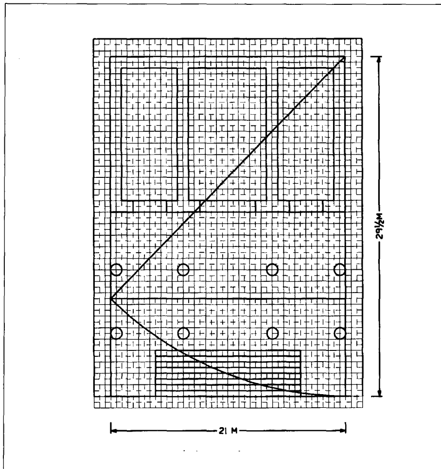
FIGURA 4: Hipotesi de restitució de la planta.
