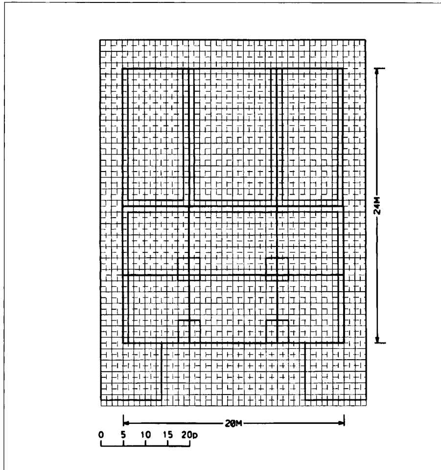
FIGURA 3: Disposicions tuscanes a nivell de fonaments.
