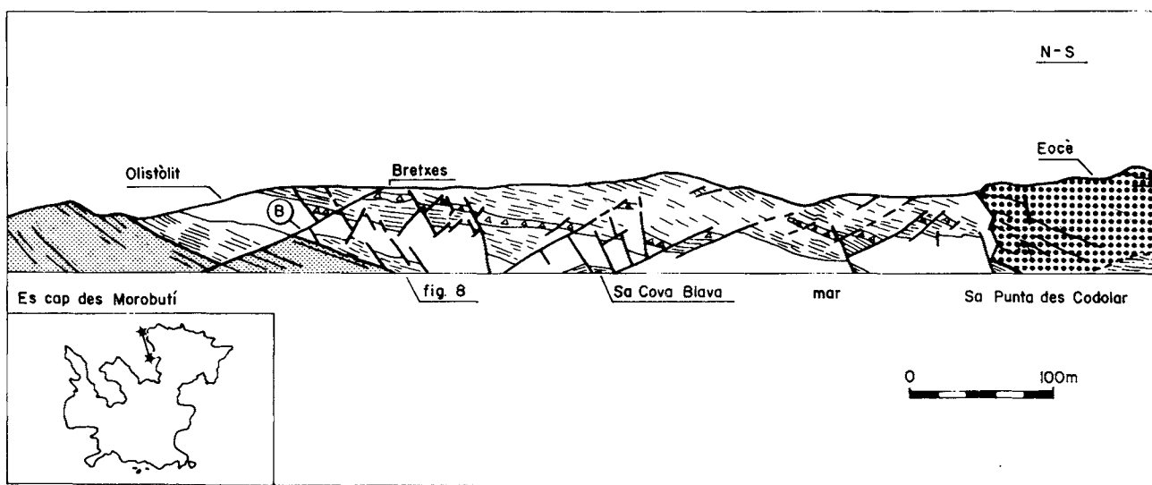
Figura 7. Penya-segat entre Es cap des Morobutí i Sa Punta des Codolar. Hi destaca el sistema de falles conjugades que tallen la sèrie mesozoica. El contacte entre el Mesozoic i l'Eocè també és per falla. Esquema realitzat a partir d'un muntatge fotogràfic. Els materials de plataforma han estat puntejats. Vegeu explicació més detallada en el text.
