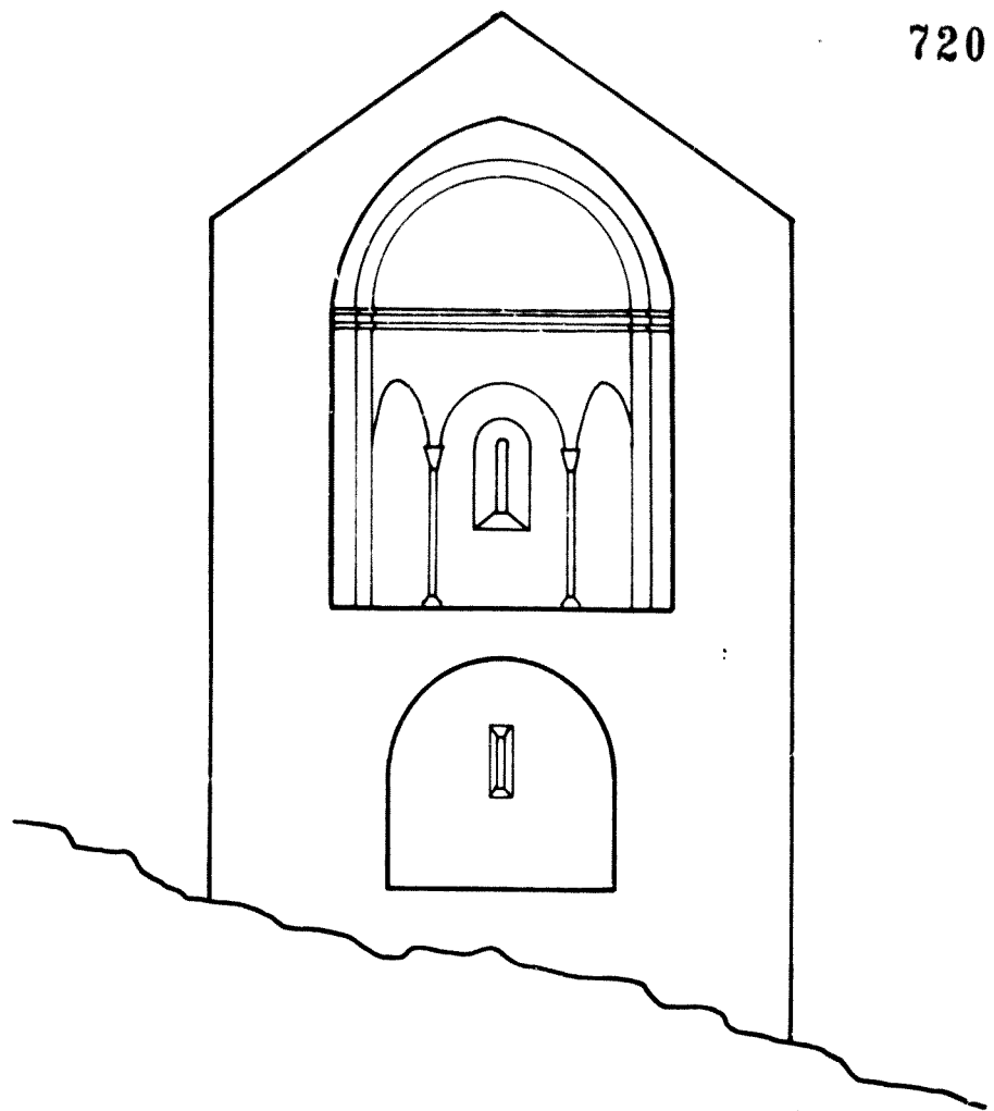
SANT MIQUEL DE MONTMAGASTRE alçat del temple romànic s. XI
