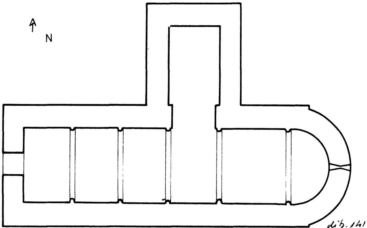
SANT MIQUEL DE COLLFRED esc. 1/100
