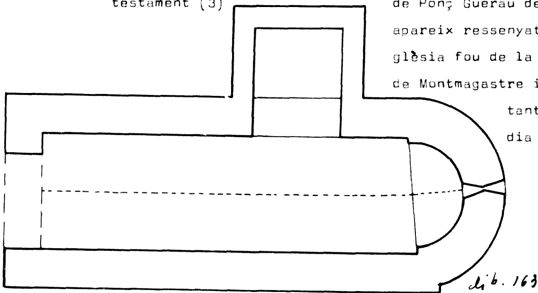
RUBIÓ VELL Església de St. Eudald esc. 1/100
