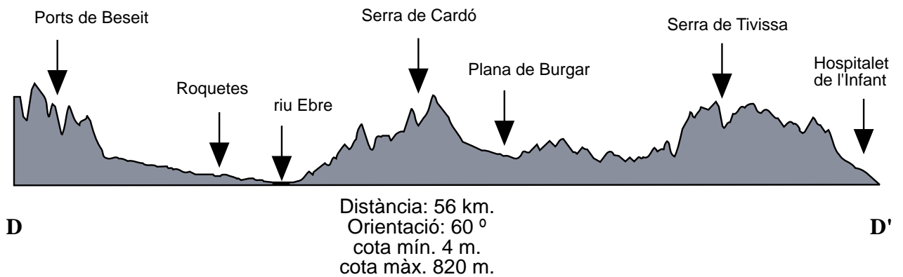
Mapa 5. Seccions topogràfiques del curs inferior de l'Ebre, indicades en el mapa 4.
