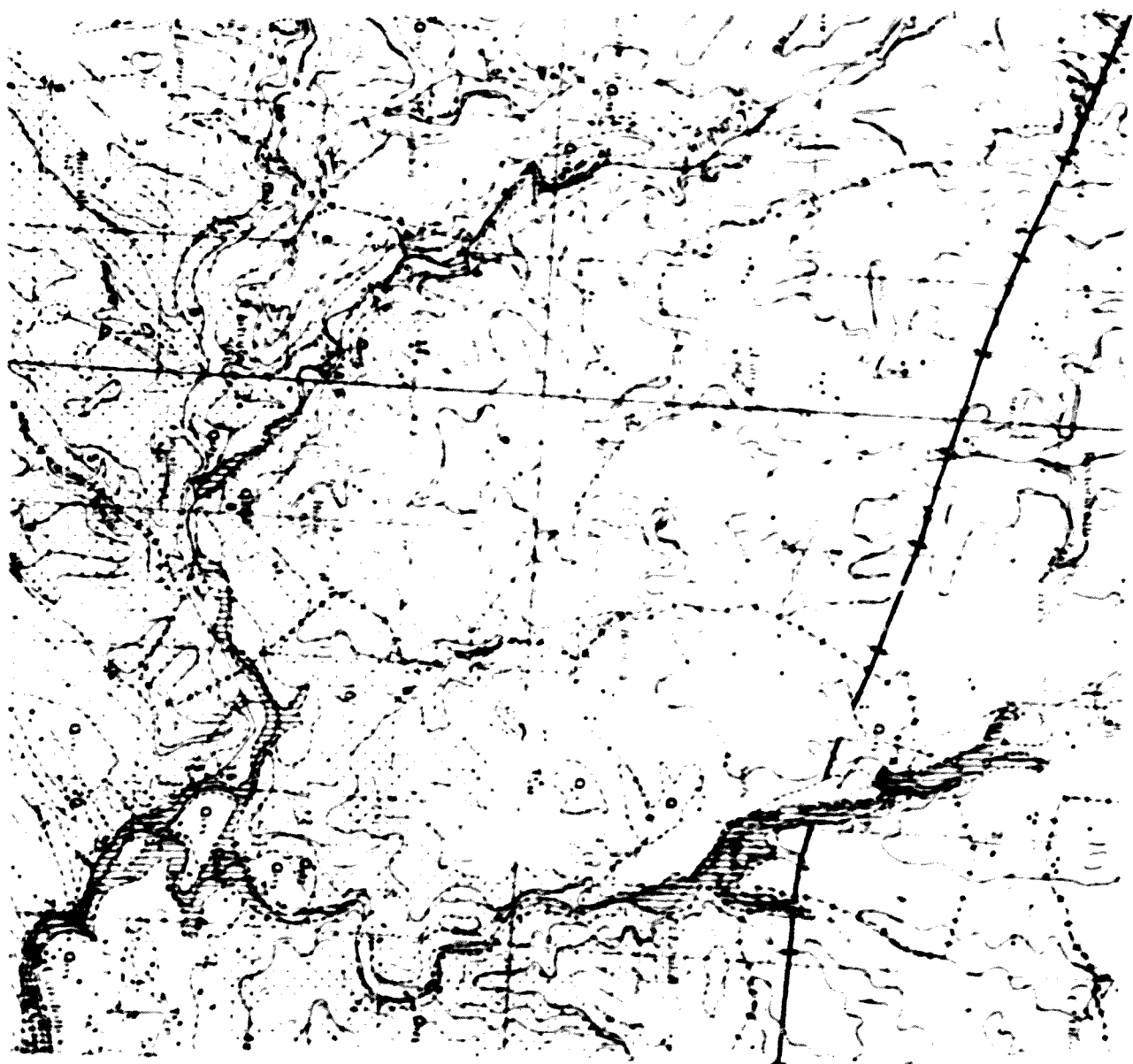
Figura 3. Mapa geologic de la zona de Linyà-Navès (extret de la fulla 330 de l'IGME, 1975) E. 1:50000.
