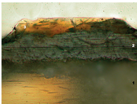
Fig. 15. Sobre la lámina metálica d'estany (capa 2) trobem l'estrat groguenc i traslúcid característic d'una corladura, d'unes 15 micres de gruix (capa 3). Microscopi òptic amb llum transmesa. Secció transversal de la micromostra núm. 1 (objectiu Mplan 50 X / 0,75). Imatge: Arte-Lab, SL / Sobre la lámina metálica de estaño (capa 2) hallamos el estrato amarillento y traslúcido característic de una corladura, de unas 15 micras de grosor (capa 3). Microscopio óptico con luz transmitida. Sección transversal de la micromuestra núm. 1 (objetivo Mplan 50 X / 0,75). Imagen: Arte-Lab, SL.
