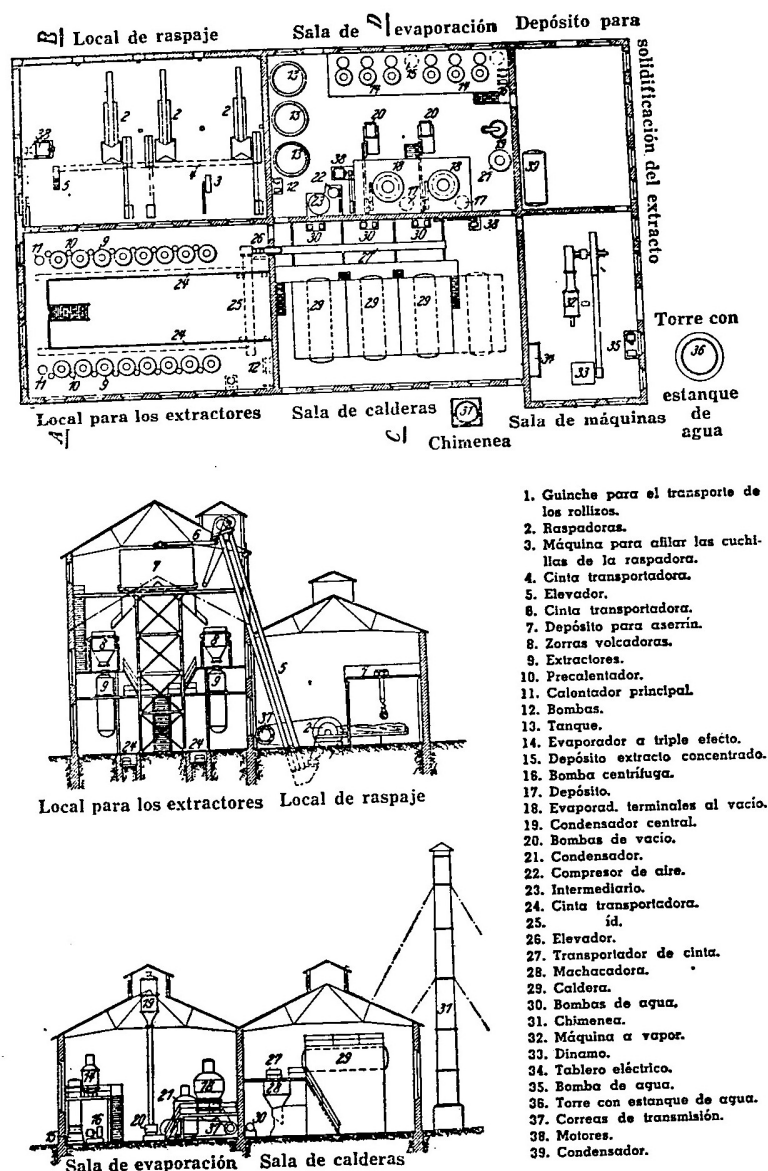
Esquema de una Fábrica de Extracto de Quebracho (Hänig).
