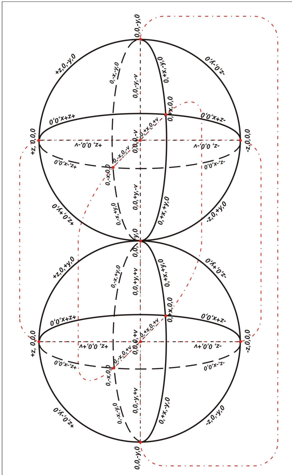
Esquema XXVI: Oscil·lació tridimensional hiperesfèrica
