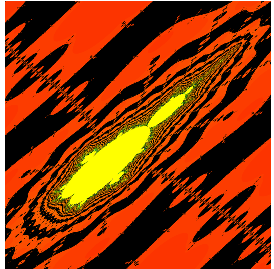
(d) A Mandelbrot-like set.
