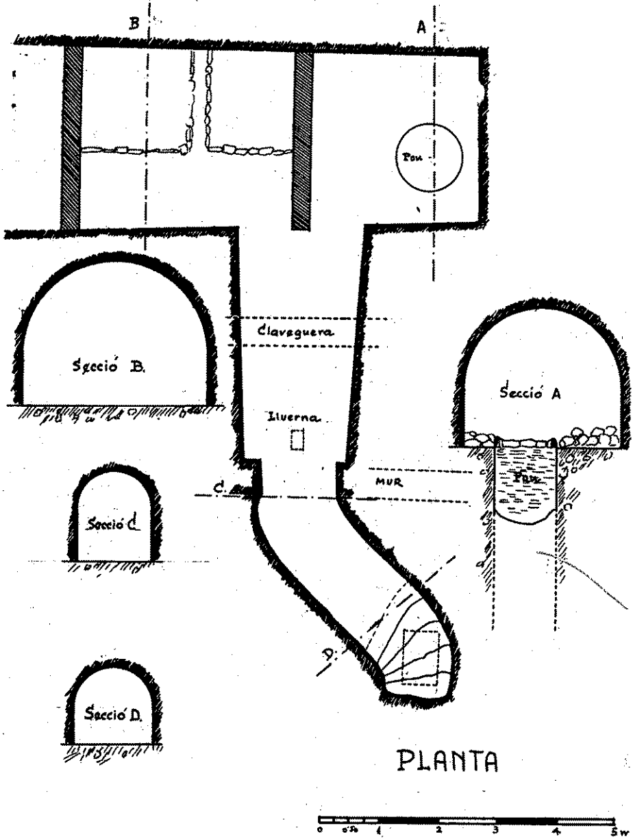
Fig. 1. Planta i seccions del soterrani de Sant Llorenç de Morunys.
