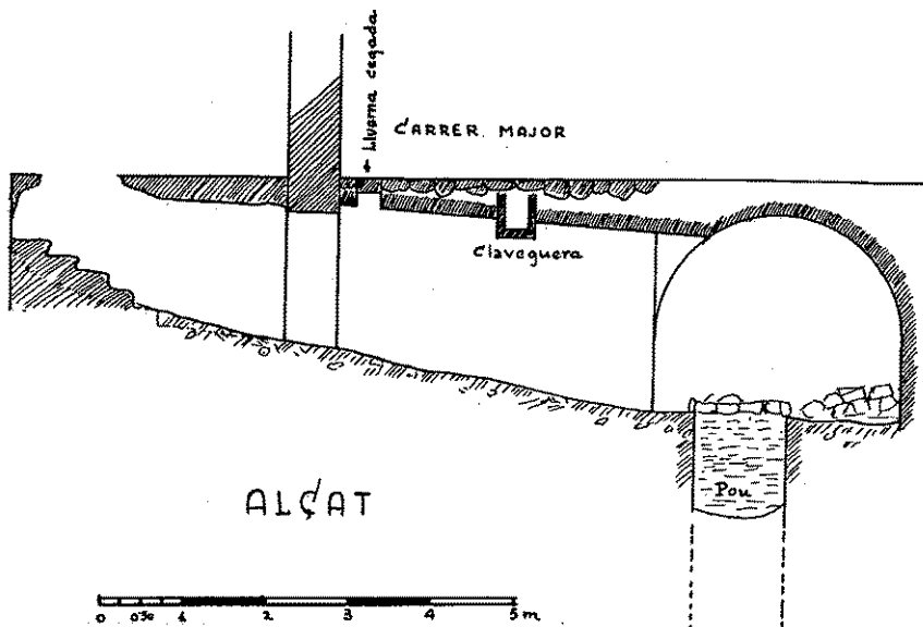
Fig. 2. Alçat del soterrani de Sant Llorenç de Morunys
