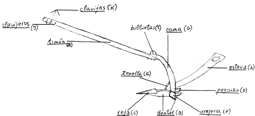
Ilustración 1. Partes del arado
