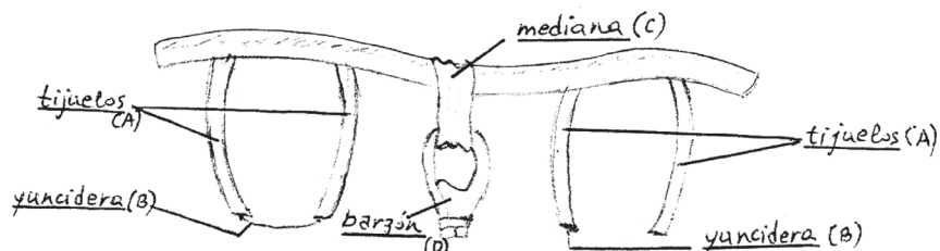
Ilustración 2. El yugo y sus partes
