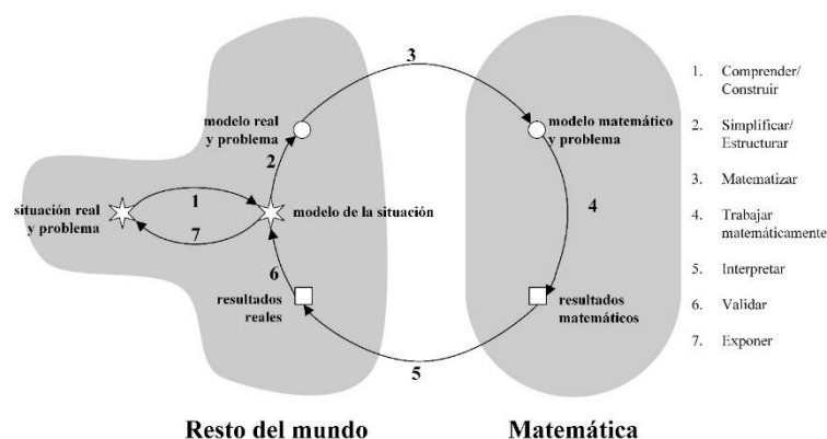
Figura 1 – Ciclo de modelización matemática Fuente: BLUM; LEIß (2007, p. 225)
